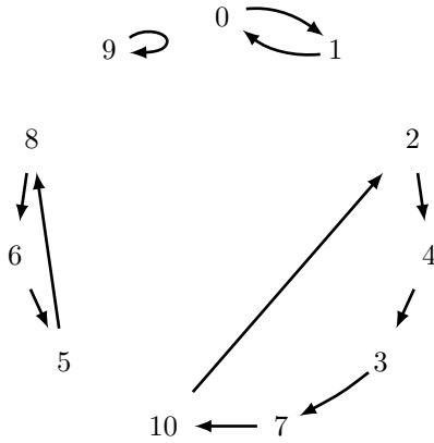
Abbildung 4.2: Der Funktionsgraph der Funktion g(x) = -x^3 + 1 \pmod{11}
