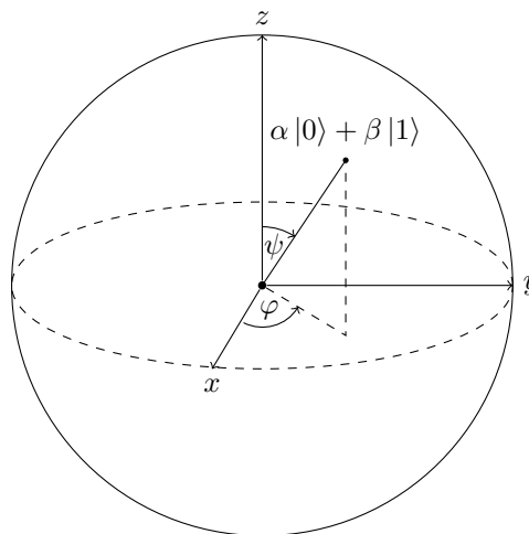
Abbildung 2.1: Die Blochkugel
